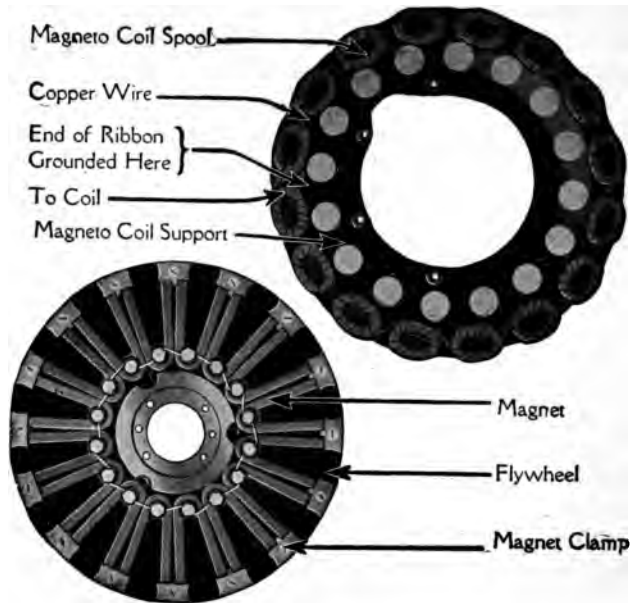
FIG. 197.—The Ford magneto.
